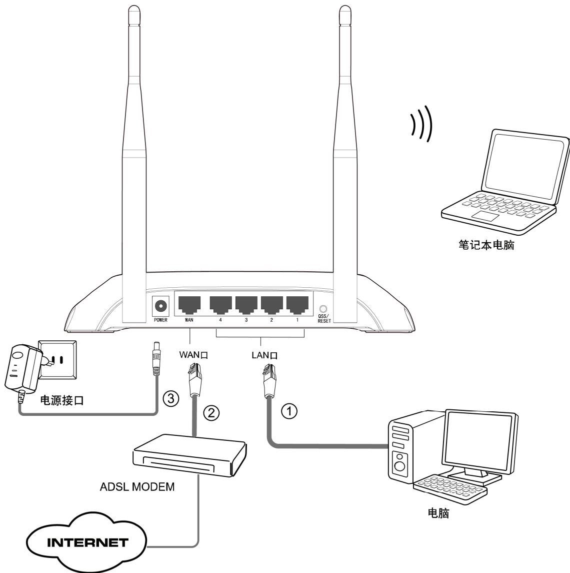
图 4-1 TL-WR841N 硬件安装示意图
